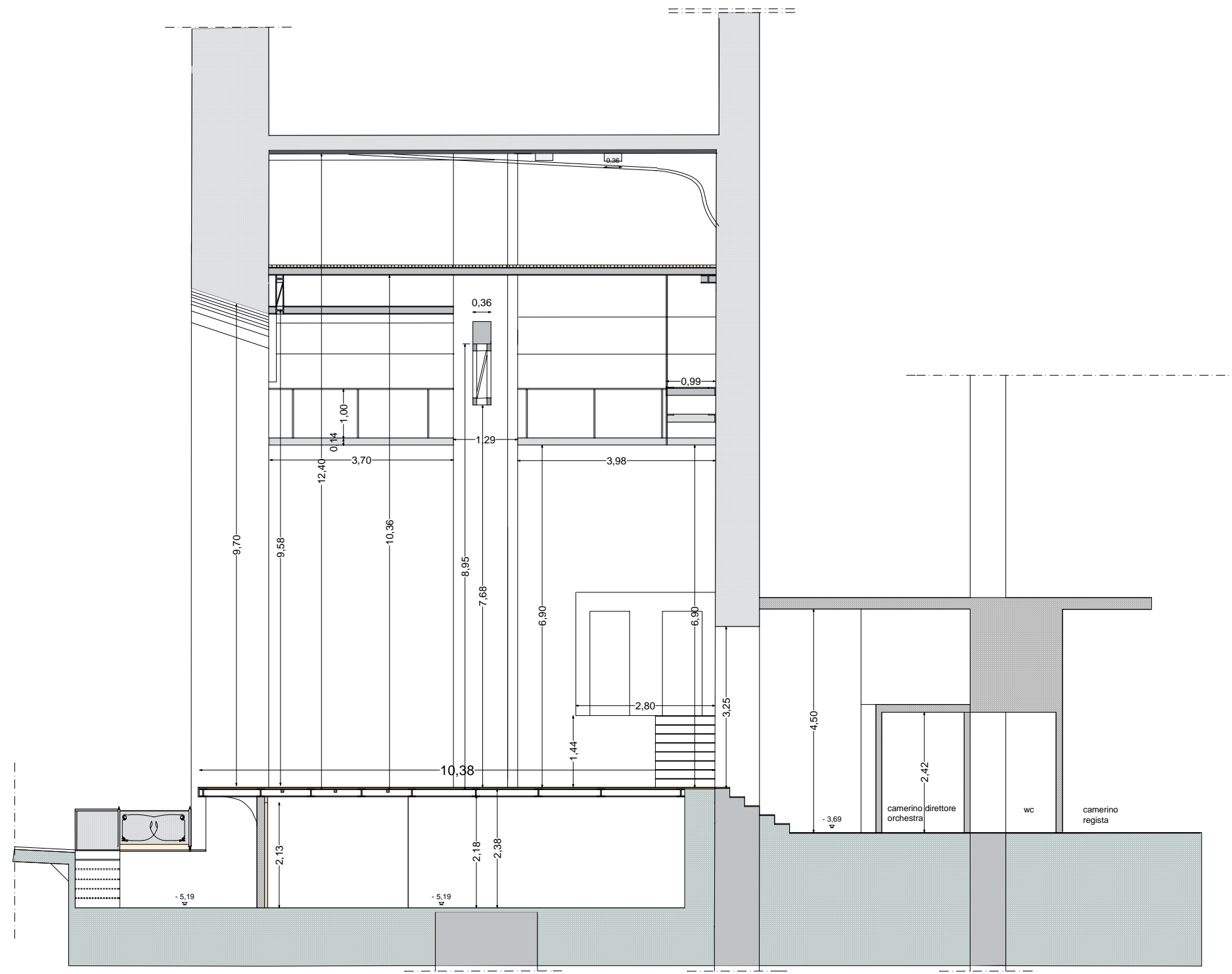
sezione longitudinale palcoscenico scala 1: 50
