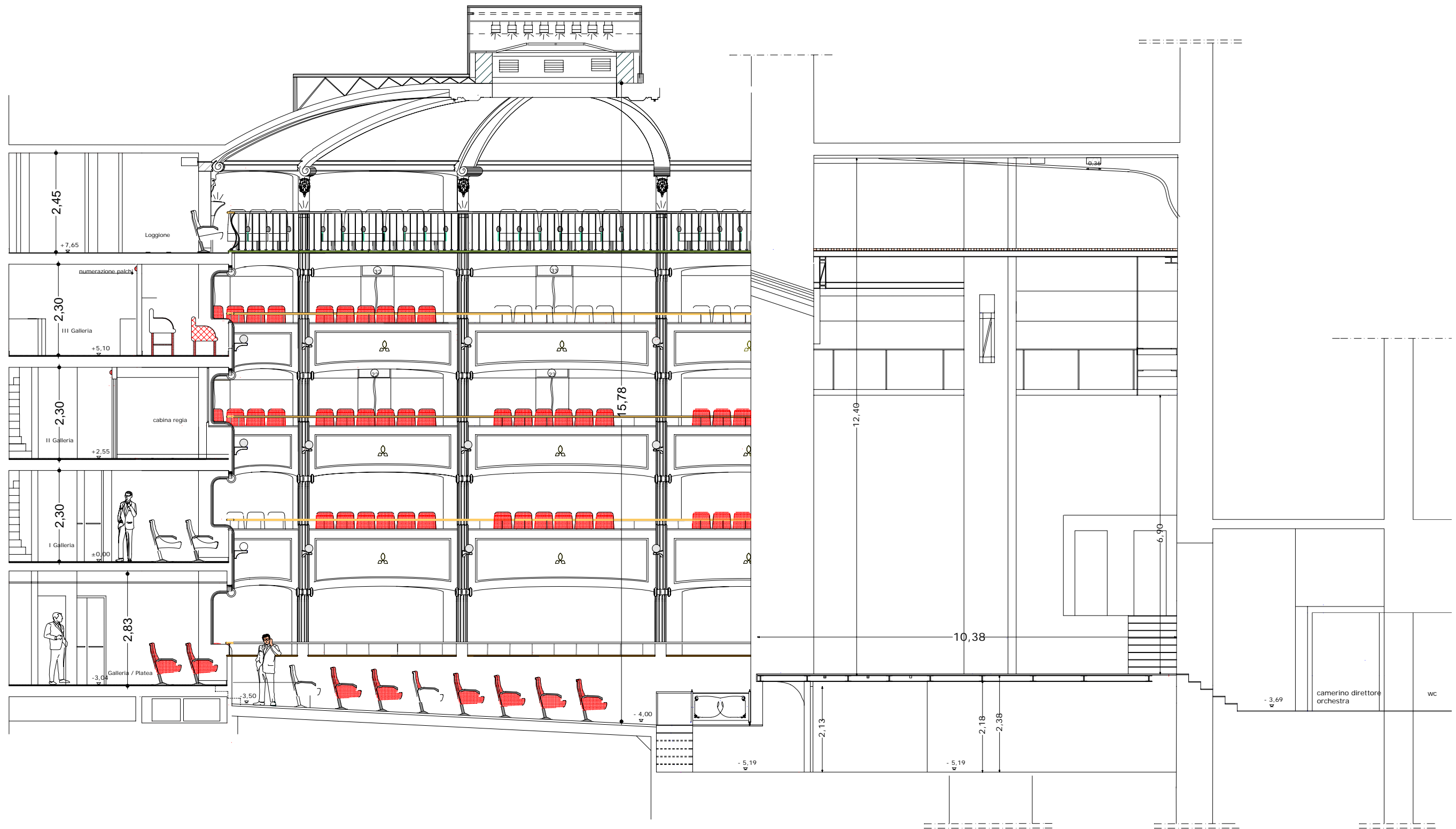
sezione longitudinale palcoscenico scala 1: 50
